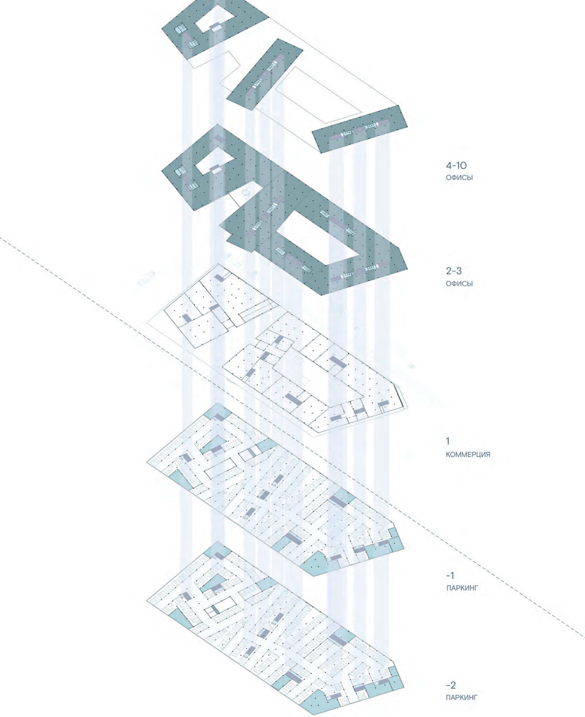
ФУНКЦИОНАЛЬНАЯ ВЗРЫВ-СХЕМА
