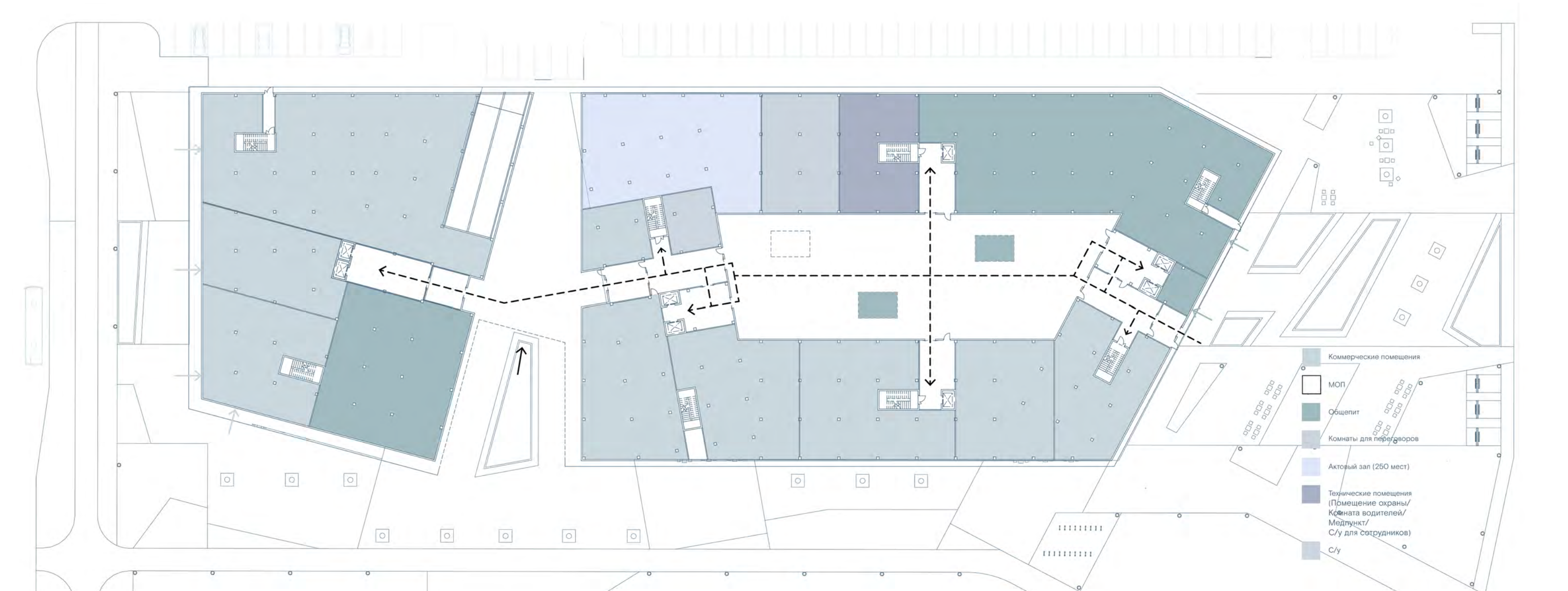
СХЕМА ПЛАНА 1 ЭТАЖА СОВМЕЩЕННАЯ С ПЛАНОМ БЛАГОУСТРОЙСТВА
