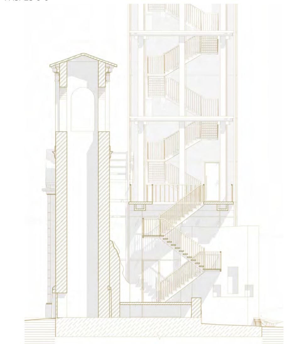
РАЗРЕЗ 3-3
