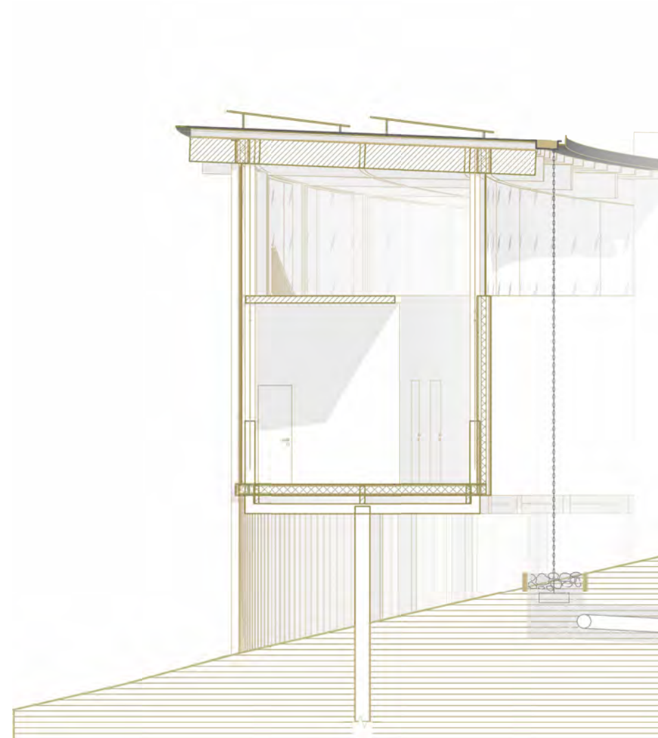
РАЗРЕЗ 3-3
