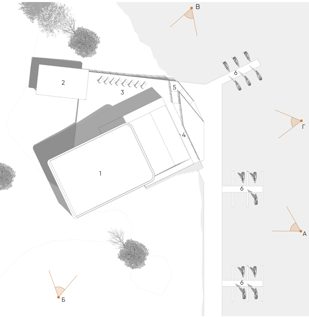
СИТУАЦИОННЫЙ ПЛАН
