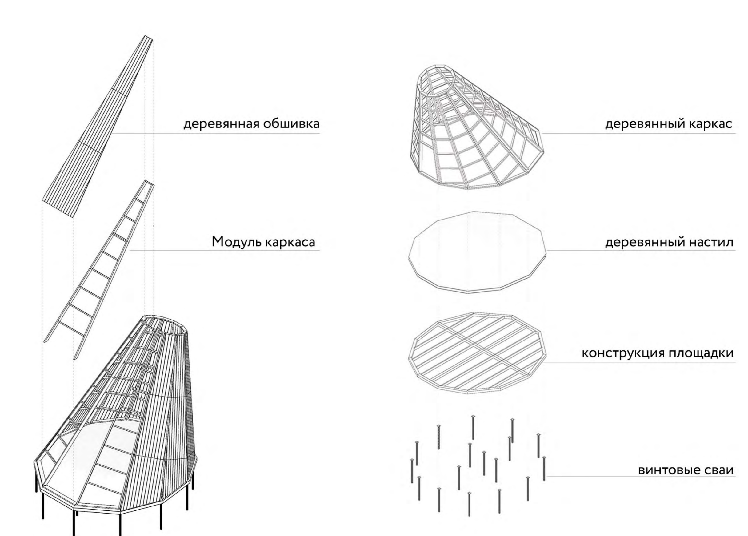
Взрыв схема 1
