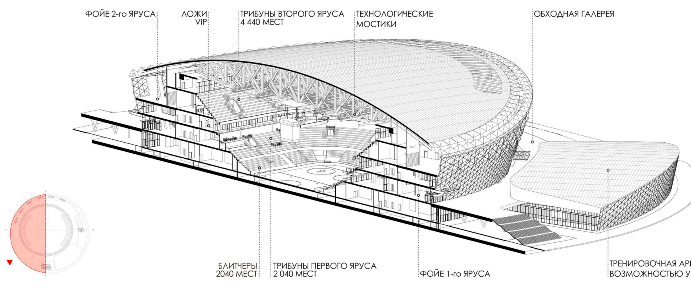
ПОПЕРЕЧНОЕ ЗО СЕЧЕНИЕ
