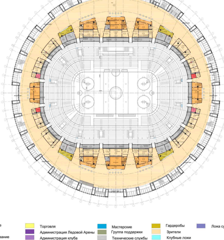
ПЛАН НА ОШМ. 14.700
