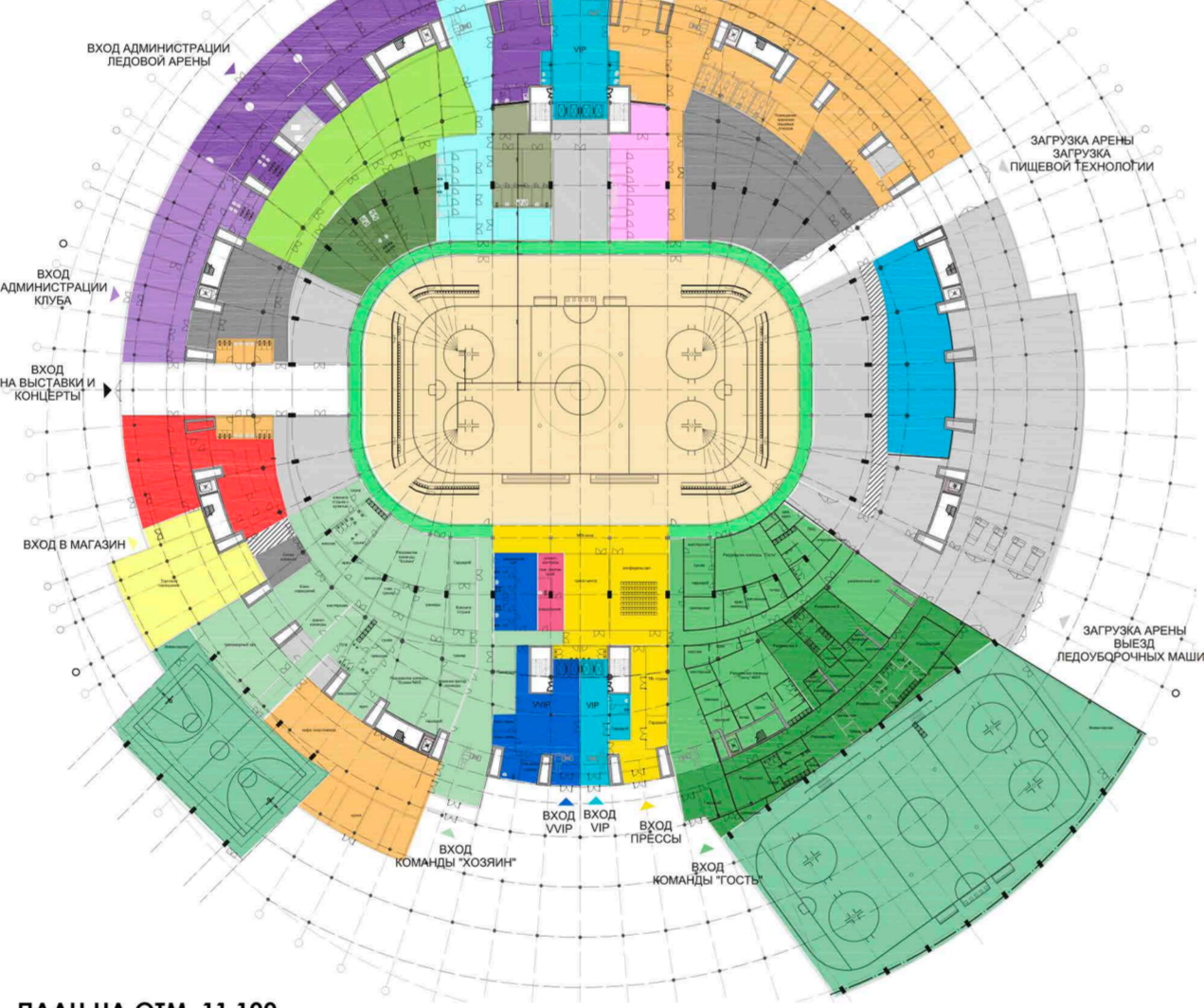
ПЛАН НА ОШМ. 11.100
