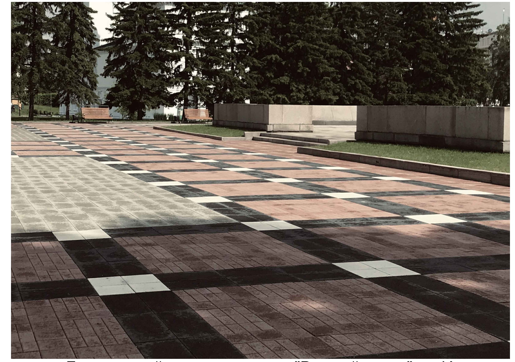
Благоустройство мемориала "Вечный огонь" в г.Иркутске
