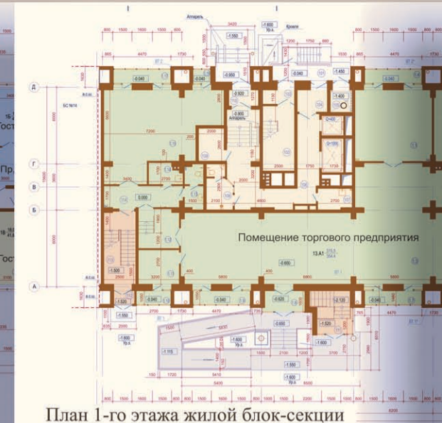
План 1-го этажа жилой блок-секции
