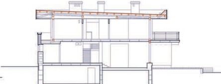
Разрез 1-1.
