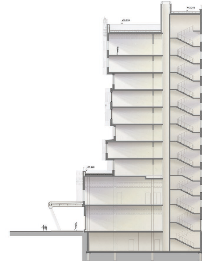
Разрез
