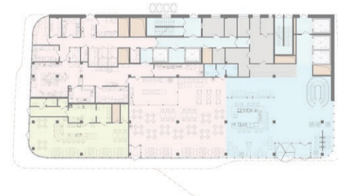
План 3 этажа
