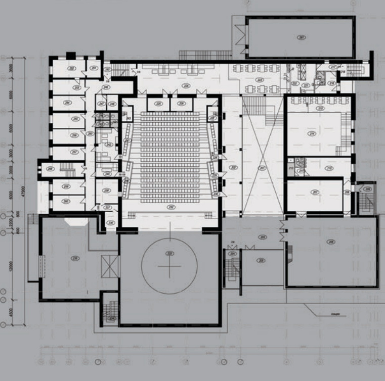
План 2 этажа
