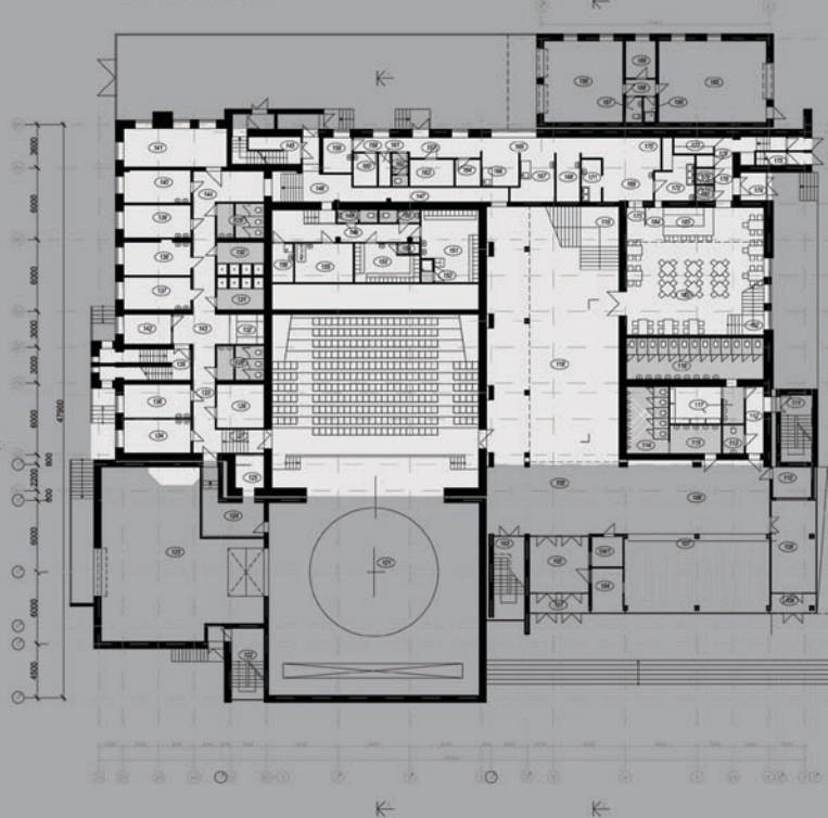
План 1 этажа
