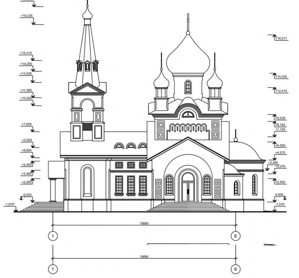
Фасад 1-6
